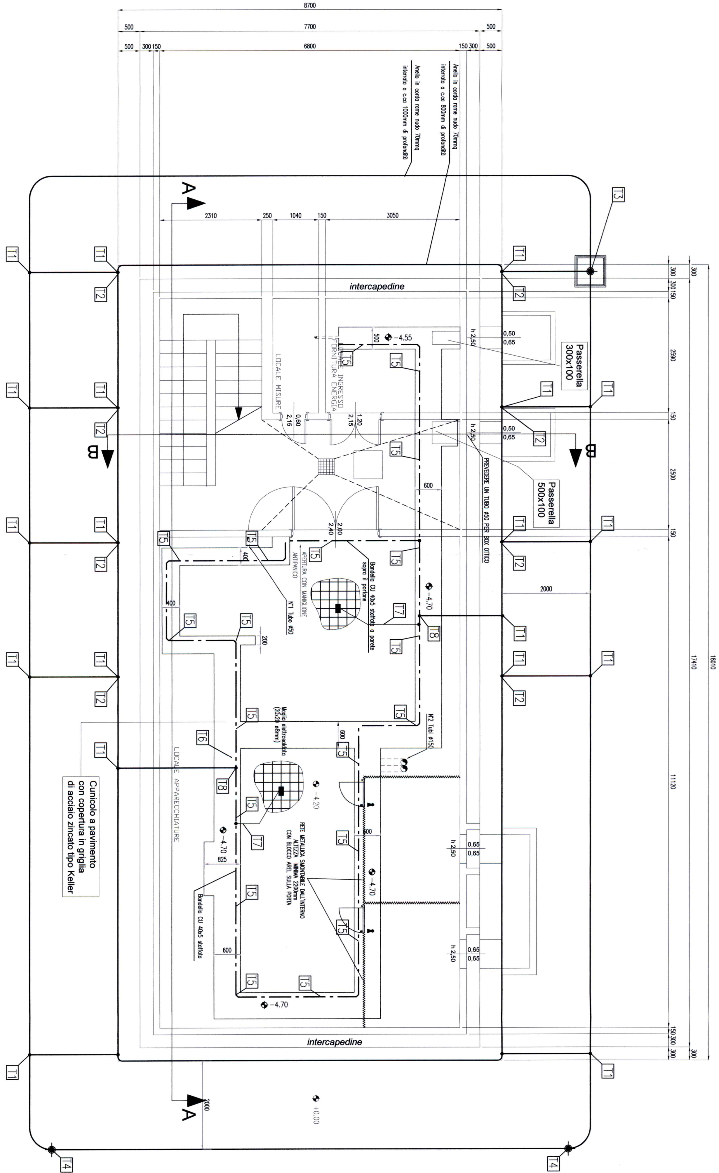
PIANTA A QUOTA -4,20
